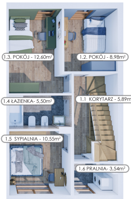
PIĘTRO
